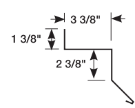
7/8" J TRIM
